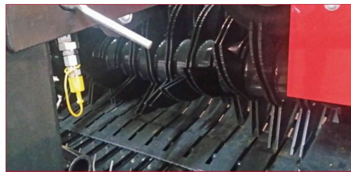
Модель RB 120 Rotor поставляется с роторным укладчиком.
